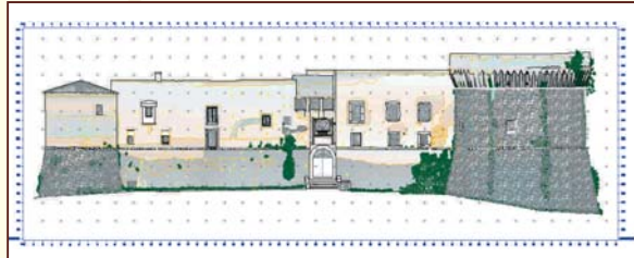
RILIEVO DEL CASTELLO ARAGONESE - CASTROVILLARI (CS)
