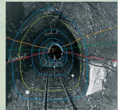
RILIEVO DELLE DEFORMAZIONI DELLA GALLERIA "STARZA" R.F.I. S.P.A. - ARIANO IRPINO (AV)
