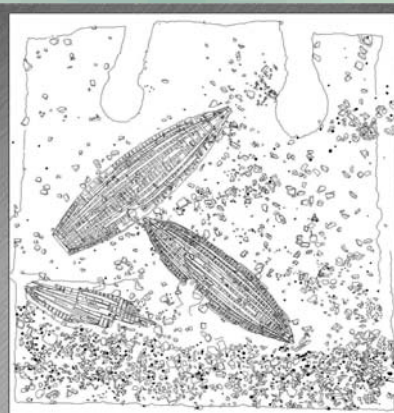
RILIEVO DEI RELITTI DI BARCHE ROMANE PIAZZA MUNICIPIO (NAPOLI) - METROPOLITANA DI NAPOLI S.P.A.
