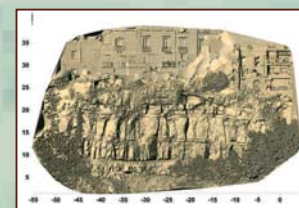
RILIEVO DEI COSTONI ROCCIOSI - R.T.P.S. - VIESTE (FG)
